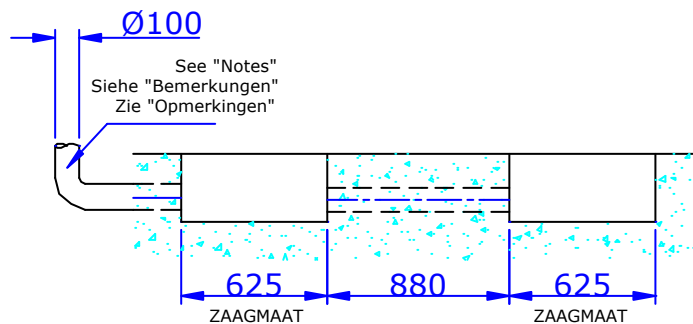
B - B
